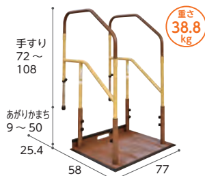
ハイタイプ両手すりBZD-03WD(N)
