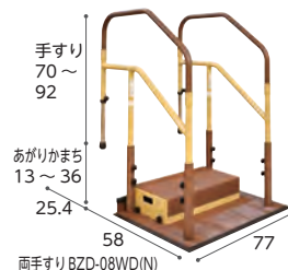
両手すり BZD-08WD(N)
