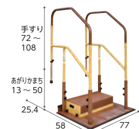
両手すり BZD-04WD(N)
