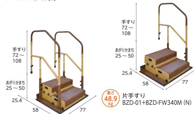
両手すり BZD-03+BZD-FW340M(N)
