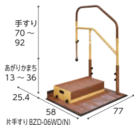
片手すり BZD-06WD(N)
